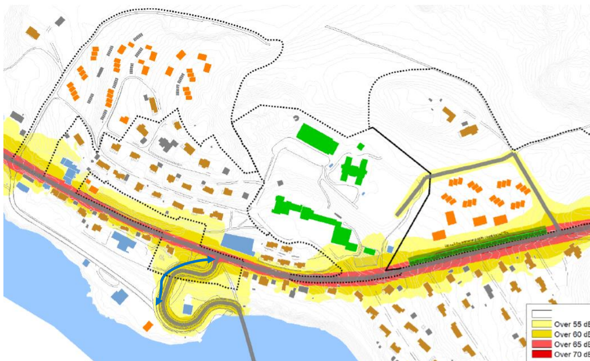
Figur 80. Støysoneskart for fremtidig situasjon med trafikk tall for 2044 med forslag til støyskjermingstiltak ved BK1. NB! Omlegging av fv. 2894 er ikke aktuelt lenger, og den delen av støykartet som er markert med blå linje er derfor heller ikke aktuell lenger.
