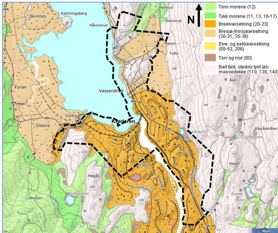
Figur 48. Løsmassekart (NGU). Omtrentlig planområde markert med svart siplet strek.
