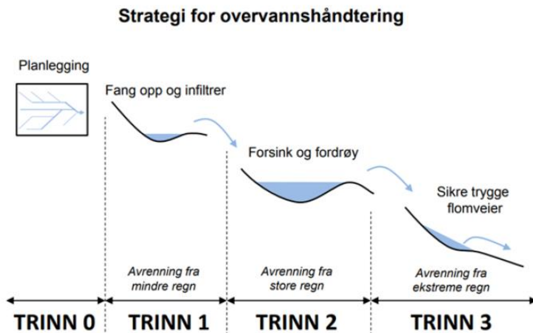
Figur 79. Prinsipp for overvannshåndtering (Norsk vann).
