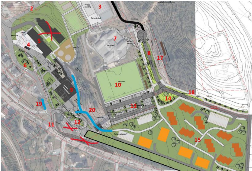
Figur 5: Snuplass for skolebusser sørøst for skolen
